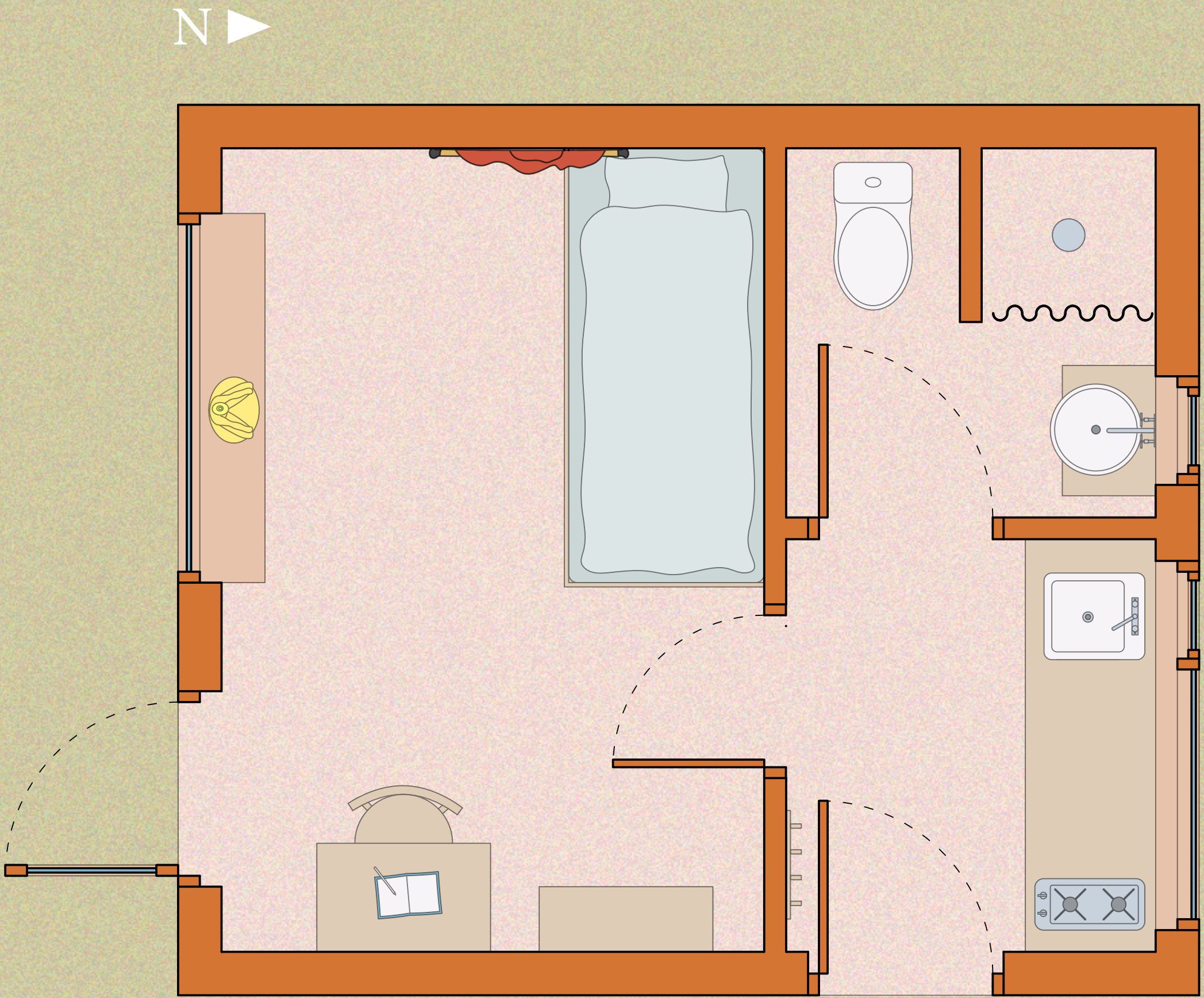
Plan 1:50
